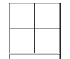
articolo 1795 contenitore 4 ante ammortizzate con piedi in metallo struttura grigio cemento piano finitura bianco statuario. 4 doors amortized cupboard with metal legs cement gray structure, top in statuary white finishing. cm. l. 136 p. 50 h. 151 colli 3 - m 3 0,29
